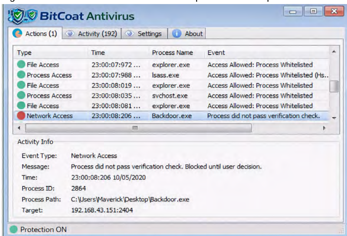
Figura 2: Bitcoat monitoriza la actividad del proceso en tiempo real
